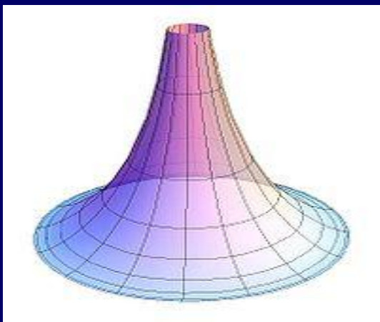
Псевдосфера
