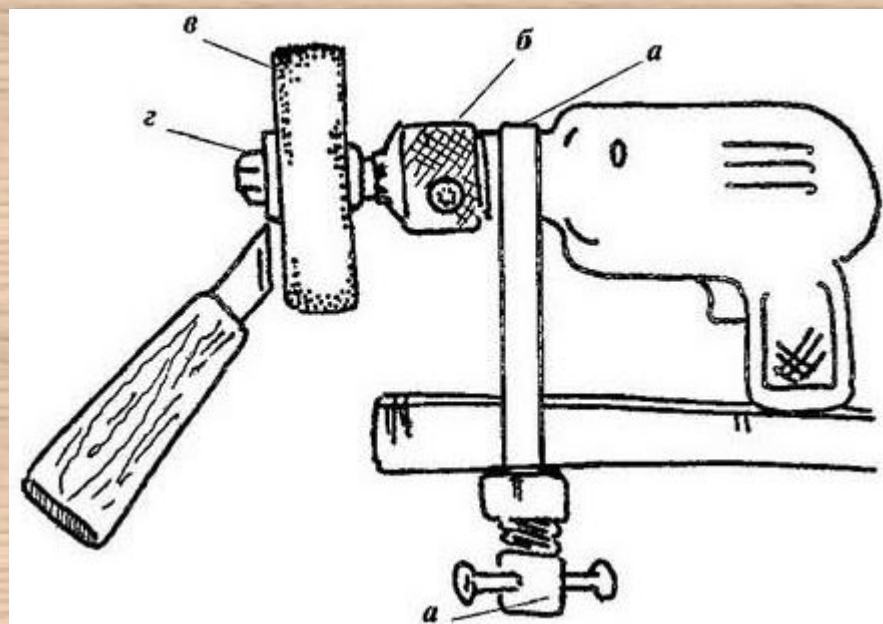
Заточка на электроточиле
