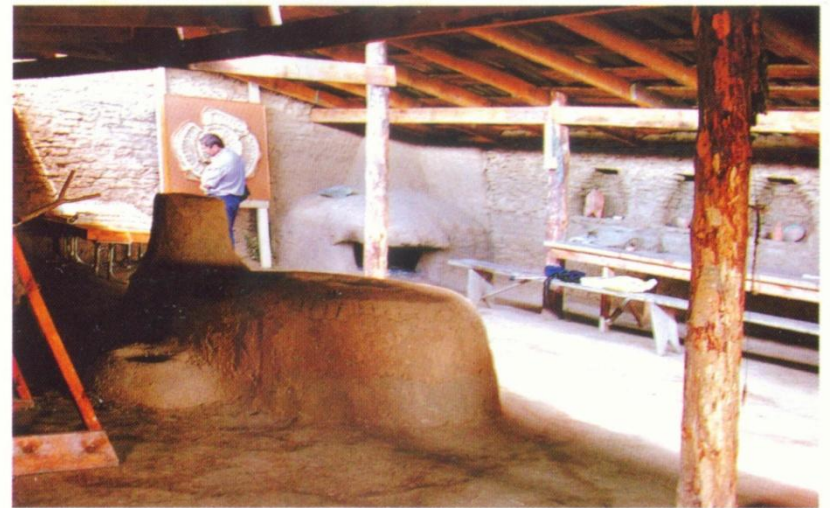
Модель архаимской печи, совмещенной с колодезем. Музей печей.
