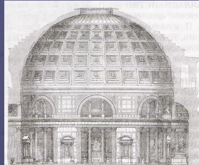
Разрез римского Пантеона. Реконструкция Адлера
