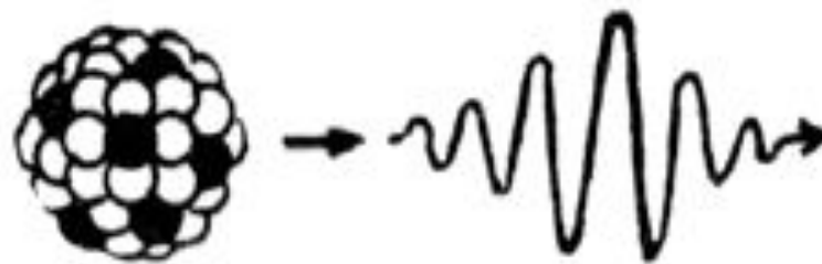
Гамма-квант
