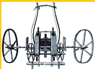
Рядовая сеялка Джетро Тулла
