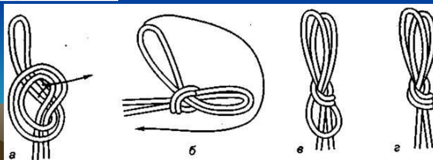
Рис. 63. «Двойной проводник»
