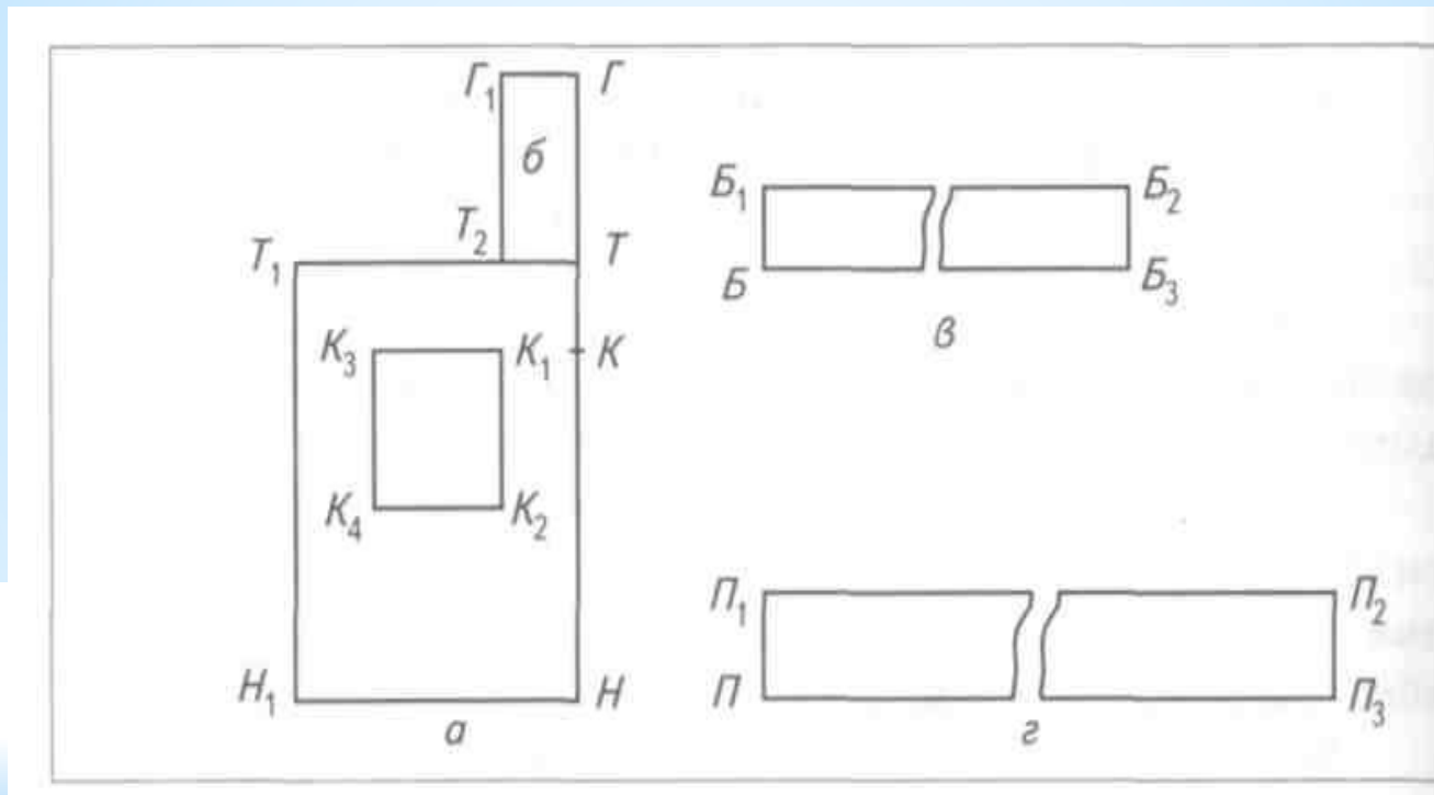
Рис. 3 Построение выкройки фартука с нагрудником: а - основная деталь фартука; б- нагрудник; в - бретель; г - пояс
