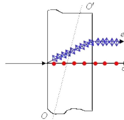
Рис. 5.15 o – обыкновенный луч, e – необыкновенный луч
