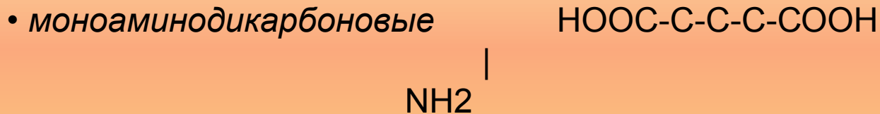
глутаминовая
