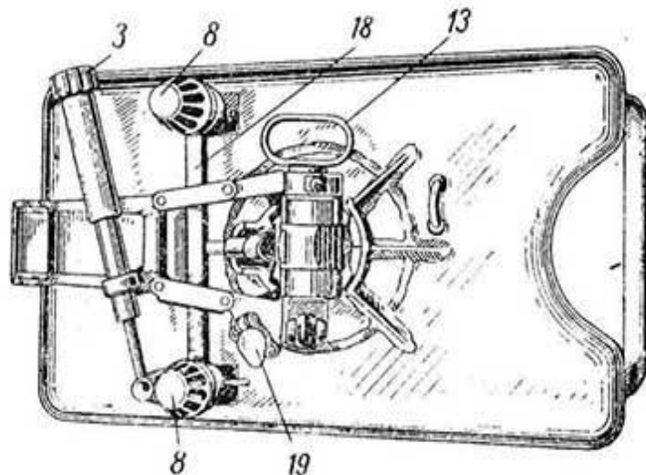
Р и с. 3. Опорная плита с горизонтирующим и поворотным механизмами:
