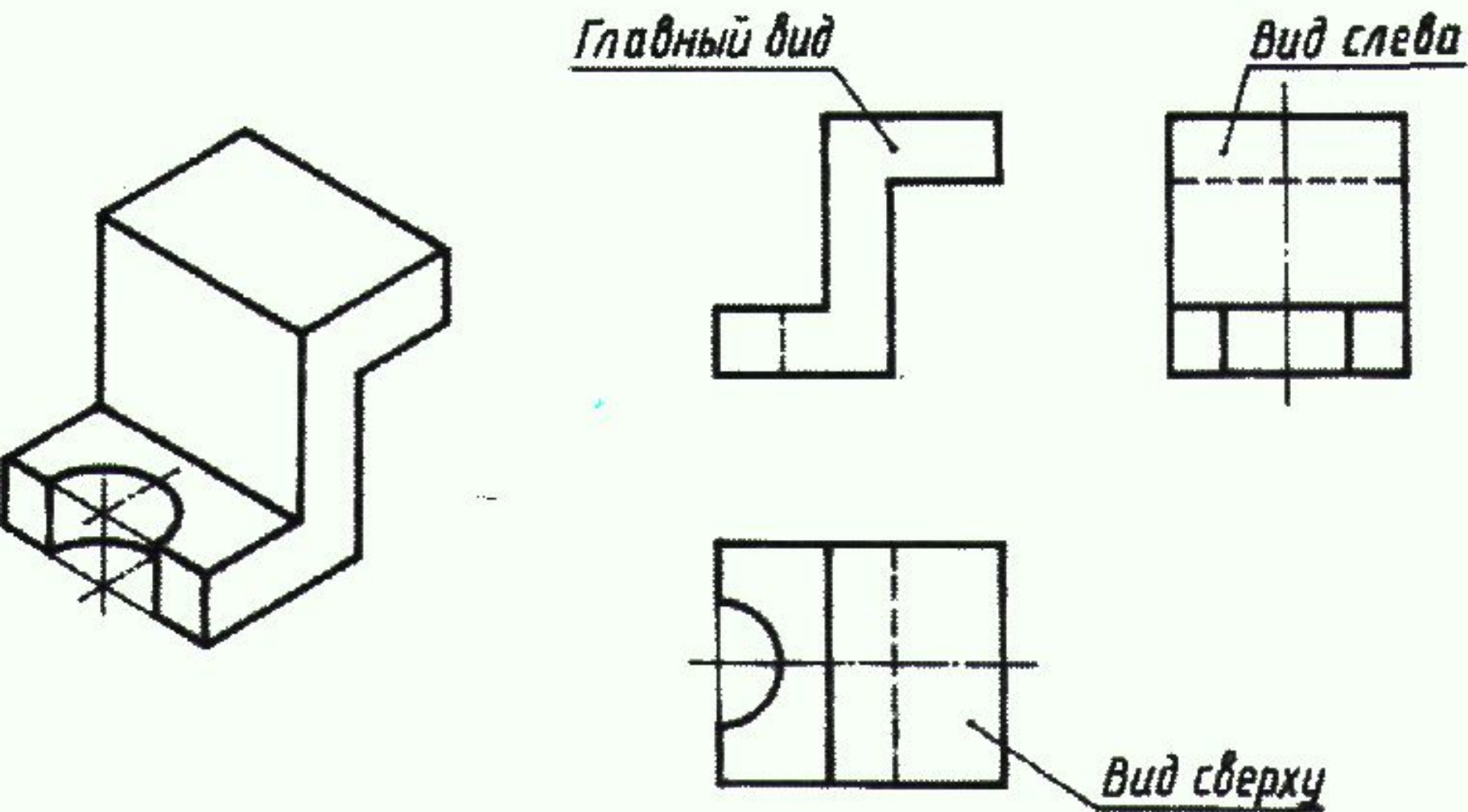
Рис. 132. Наглядное изображение и чертеж детали
