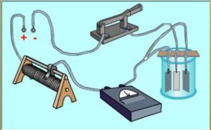
Электрическая проводимость веществ
