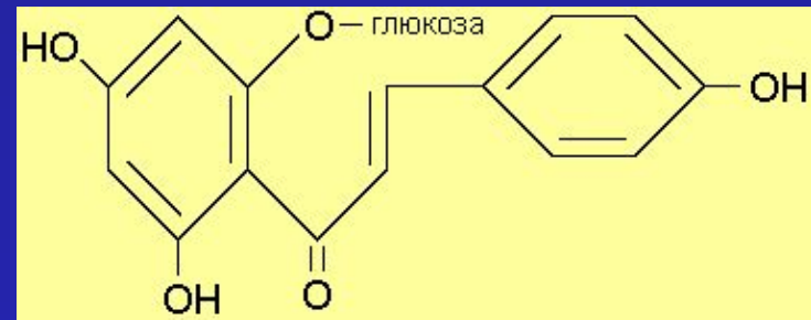
Изосалипурпозид
