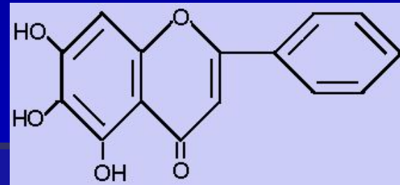
байкалеин
