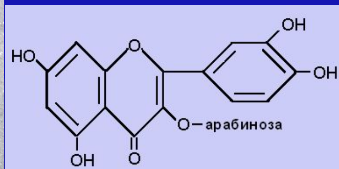
авикулярин
