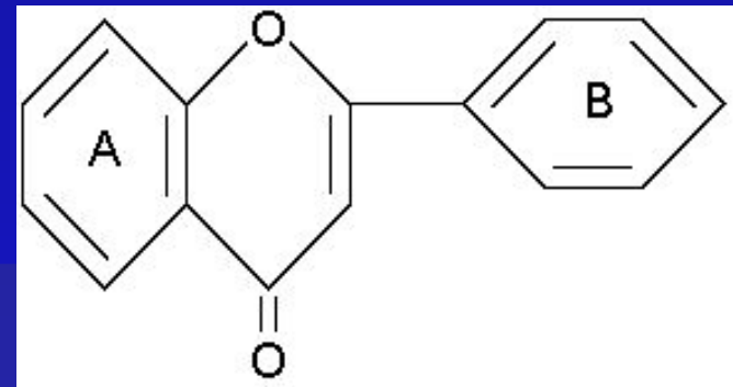
2-фенилбензо-γ-пирона (флавона).
