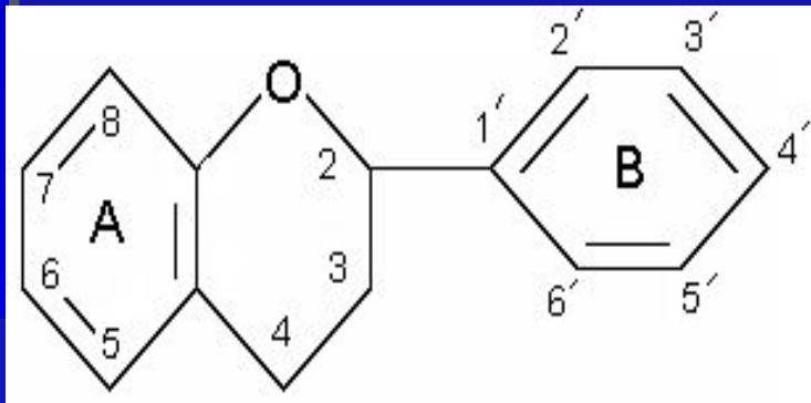
2-фенилбензопирана (флавана)
