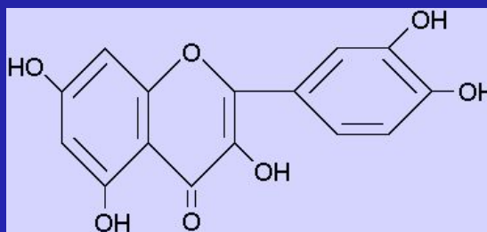
кверцетин
