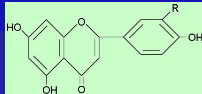
Лютеолин R=OH
