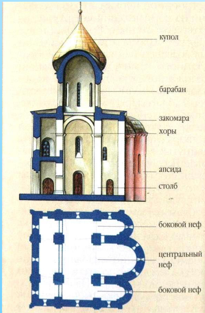
схема крестово-купольного храма
