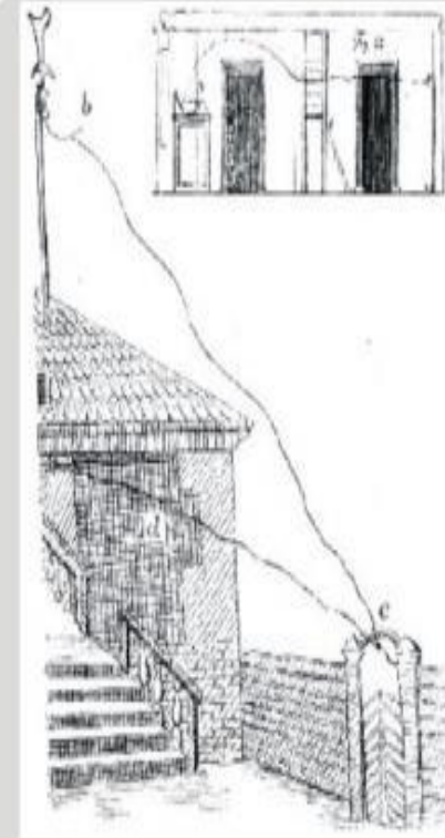
Прообраз электроскопа «указатель электрический». Проводник соединял линейку с железным прутом на крыше, притягивавшим атмосферное электричество. Рисунок М.В.Ломоносова и Г. В. Рихмана.
