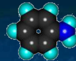
модель молекулы
