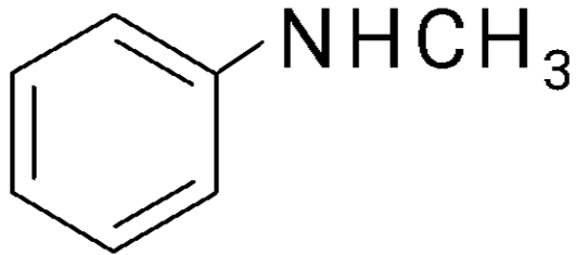
N-Метиланилин (вторичный амин)
