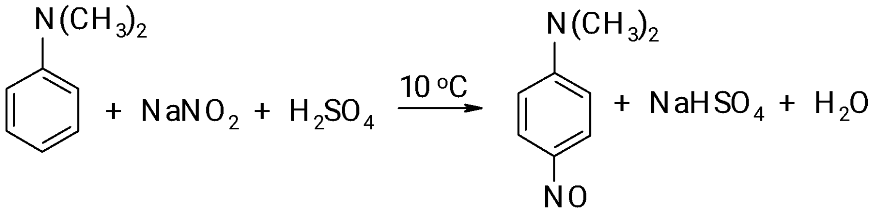
p-Нитрозо-N,N-диметиланилин
