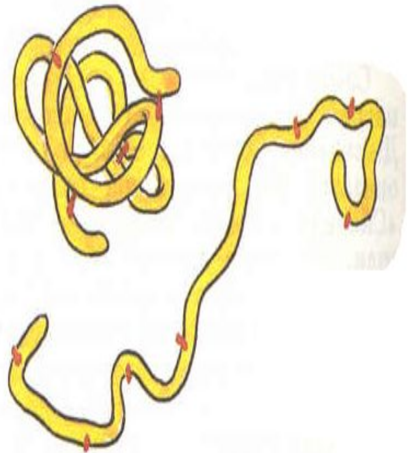
Денатурация молекулы белка.
