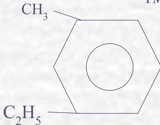
1 метил 3 этилбензол
