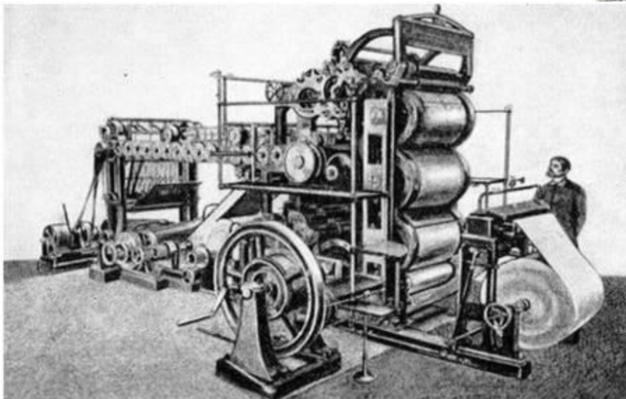
Друкарський верстат
