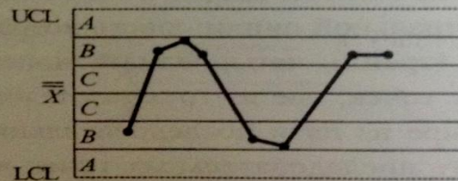
Рис. 4.3. Критерии особых причин на карте Шухарта:
