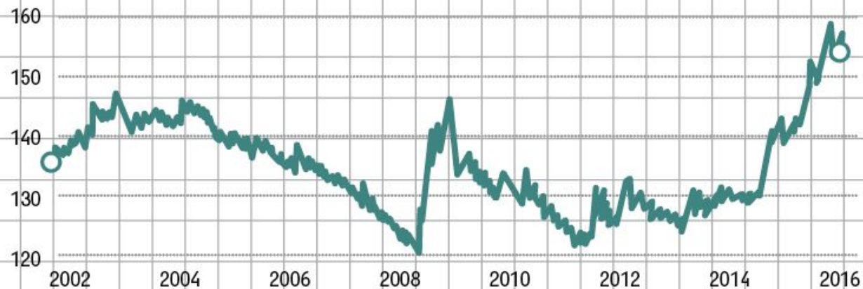
Что происходит с акциями
