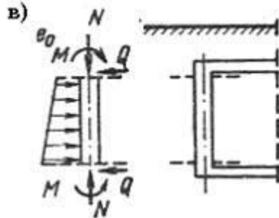
Рис. 12.1. Сжатые элементы
