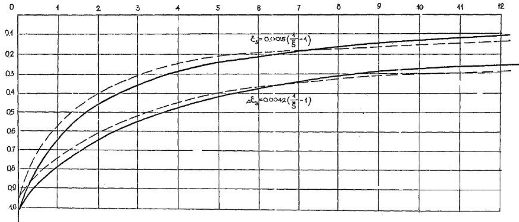
Рисунок 7. Зависимость приращений деформаций арматуры \Delta \epsilon_s от высоты сжатой зоны \xi
