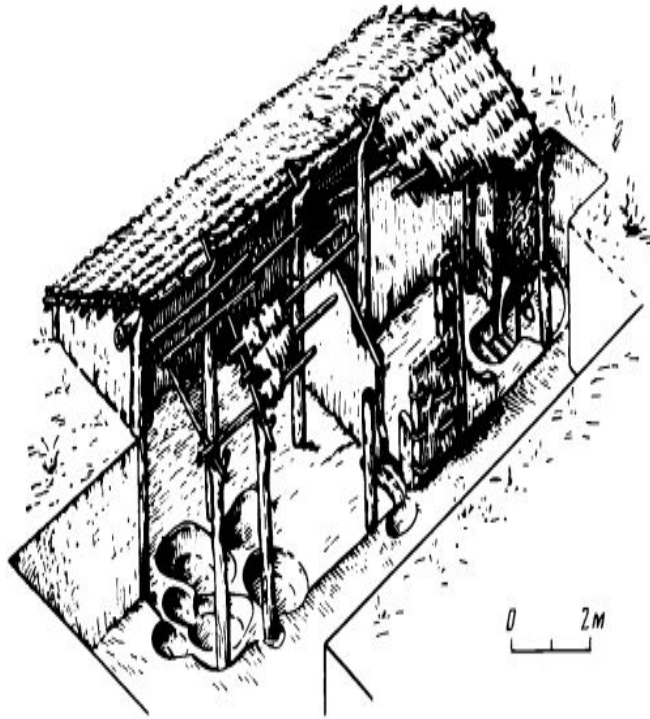
Рис. 1. Строительный комплекс 7 первой половины IV в. до н. э. Реконструкция К. К. Марченко
