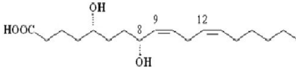
psiCa
