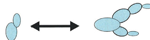
filamentous form
