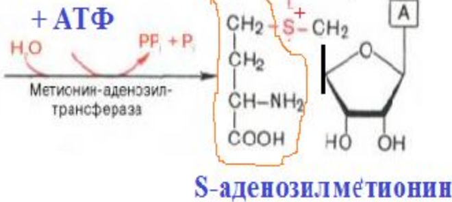
Метионин
