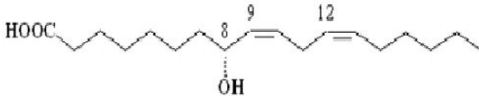
psiBa
