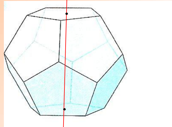
Додекаэдр
