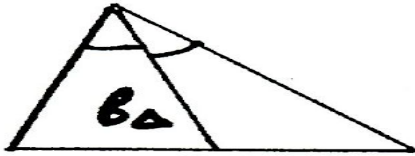
биссектриса
