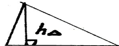
высота
