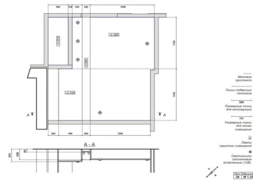
Конструкция подвесного потолка в сан. узле. Размеры на конструкции.
