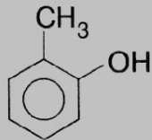
2-метилфенол (орто-крезол)
