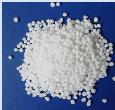
Аммиачная селитра
