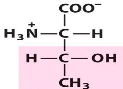
Треонин (Thr)
