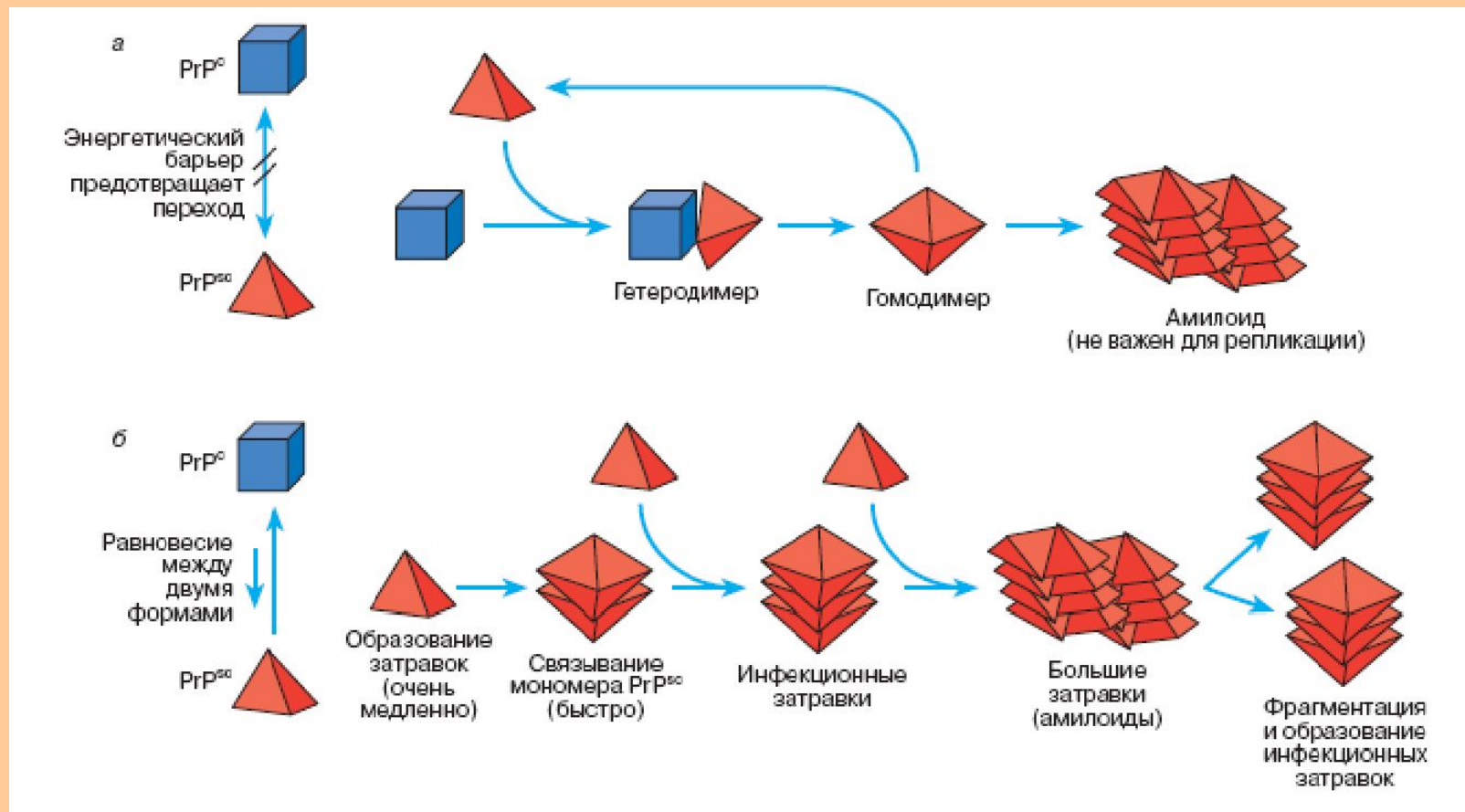
Рис. 2. Модели превращения нормально свернутого в основном \alpha -спирального приона ( \text{PrP}^c ) в неправильно свернутый в основном \beta -складчатый \text{PrP}^{sc} , а – модель плохого шаблона. \text{PrP}^{sc} связывается с \text{PrP}^c и навязывает ему неправильную структуру; б – модель затравок-зародышей. Редко образующаяся форма \text{PrP}^{sc} может образовывать затравки-зародыши, которые связывают все образующиеся молекулы \text{PrP}^{sc} и поэтому сдвигают равновесие между \text{PrP}^c и \text{PrP}^{sc} в сторону последней (no: Aguzzi A., Polymeridou M. Mammalian prion biology: One century of evolving concepts // Cell. 2004. Vol. 116. P. 313–327)
