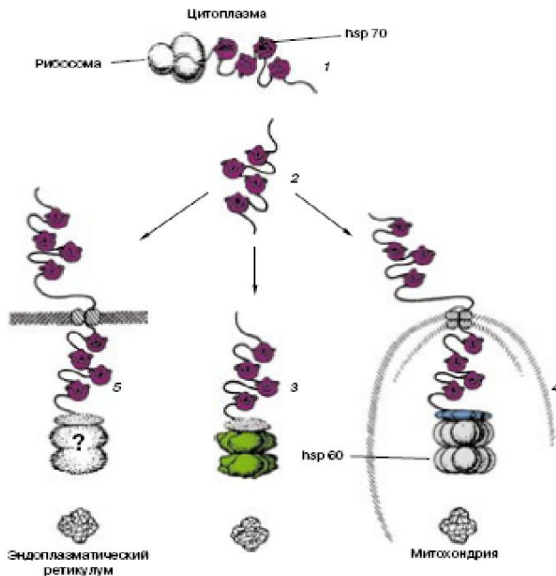
Рис. 4. Схема, показывающая участие шаперонов и шаперонина в сворачивании белка в клетке эукариот. 1 – Сходящая с рибосомы полипептидная цепь, связанная с шаперонами hsp70 цитоплазмы; 2 – шапероны hsp70 акранируют гидрофобные области полипептида, предотвращая его агрегацию; 3 – белки, сворачивающиеся в цитоплазме, передаются с шаперона hsp70 на цитоплазматический шаперонин, где и происходит сворачивание; 4 – белки, сворачивающиеся в митохондриях. Цитоплазматический шаперон hsp70 "подносит" развернутый белок к внешней мембране митохондрии. Митохондриальный шаперон hsp70, прочно связываясь с пересекающим мембрану белком, способствует его "втягиванию" внутрь митохондрии, а затем передает его на митохондриальный шаперонин, где и происходит сворачивание; 5 – белки, сворачивающиеся в эндоплазматическом ретикулуме. Цитоплазматический шаперон hsp70, с одной стороны, и шаперон hsp70 просвета эндоплазматического ретикулума, с другой, обеспечивают проникновение развернутого белка через мембрану. Детали сворачивания таких белков пока не выяснены.
