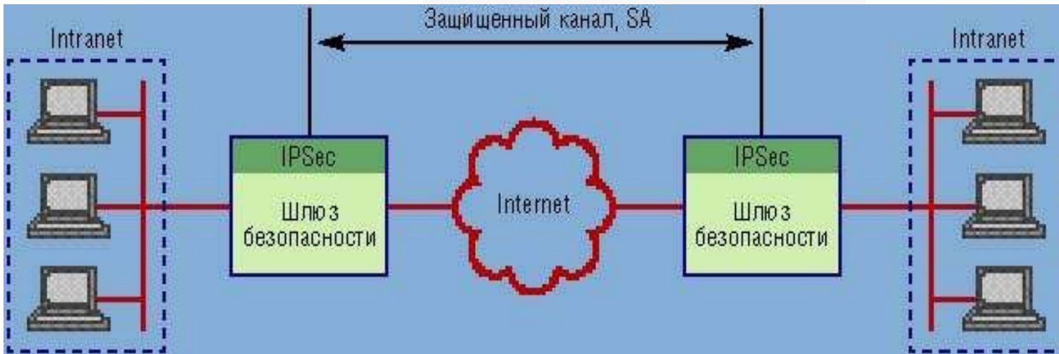
Схема «шлюз-шлюз».
