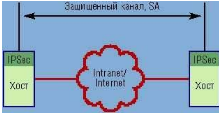
Схема «хост-хост».
