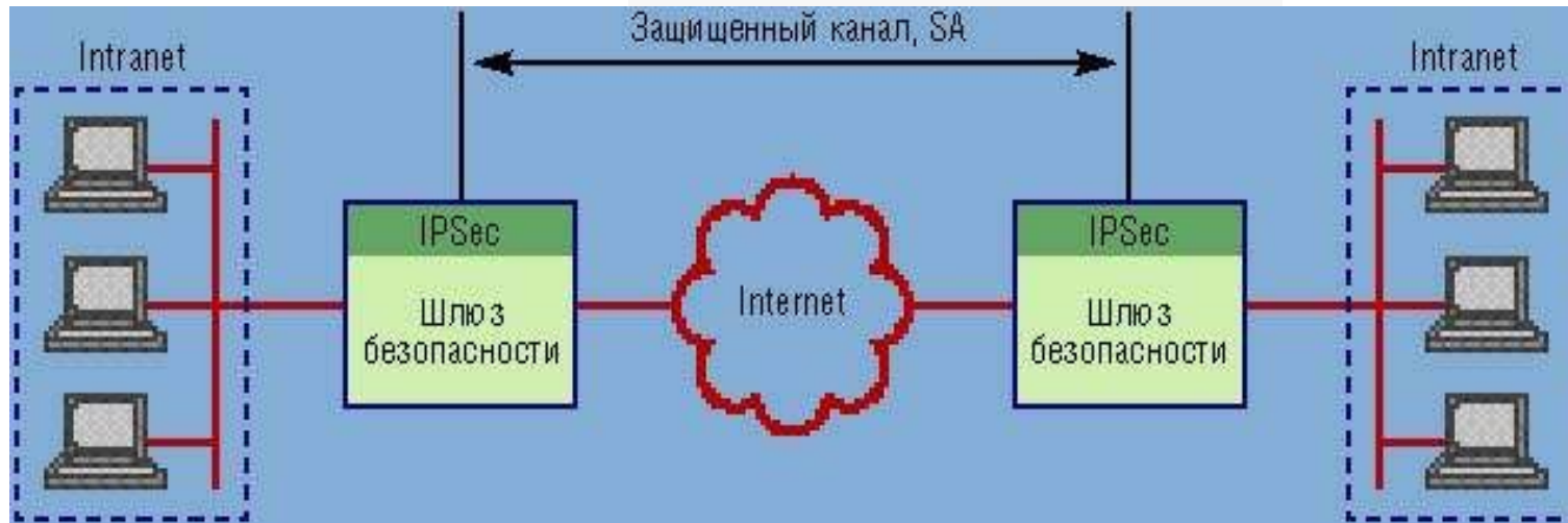
Схема «шлюз-шлюз».
