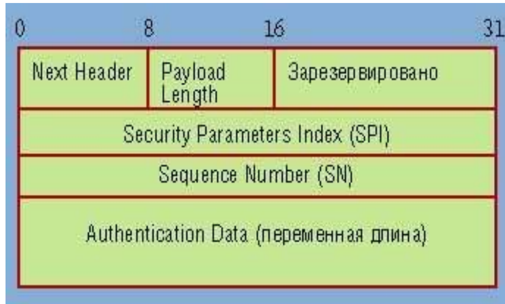
Структура заголовка протокола AH
