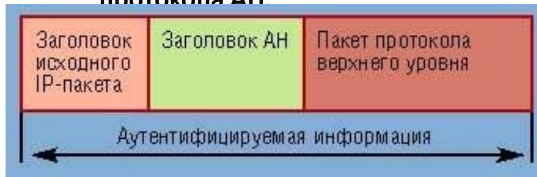
Результирующий пакет протокола AH в транспортном режиме.
