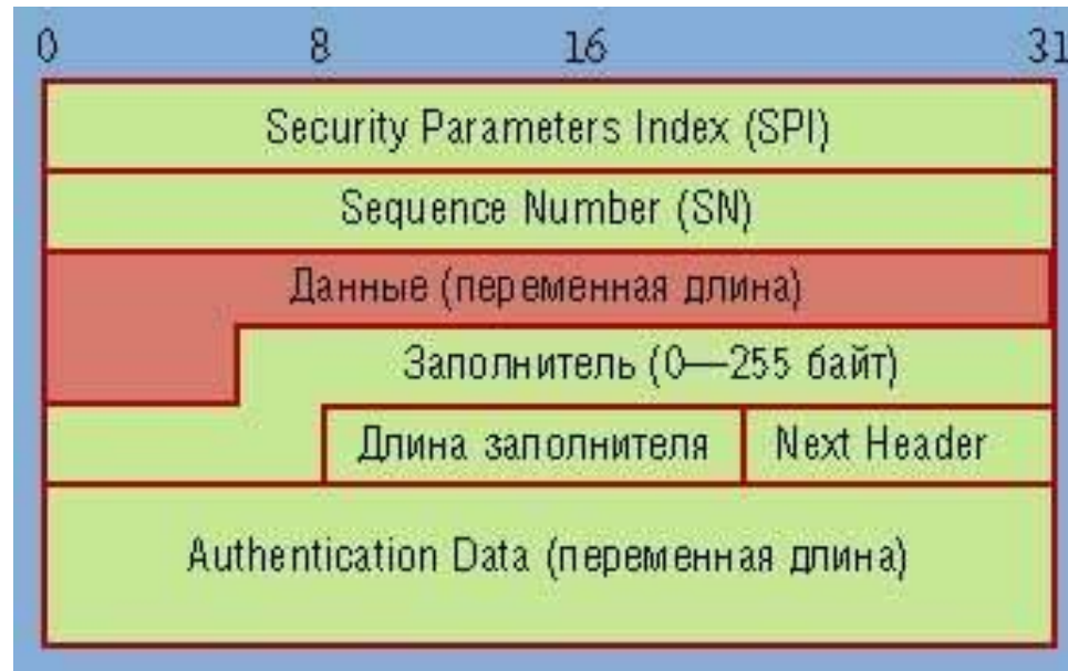
Структура заголовка протокола ESP.
