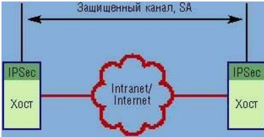
Схема «хост-хост».
