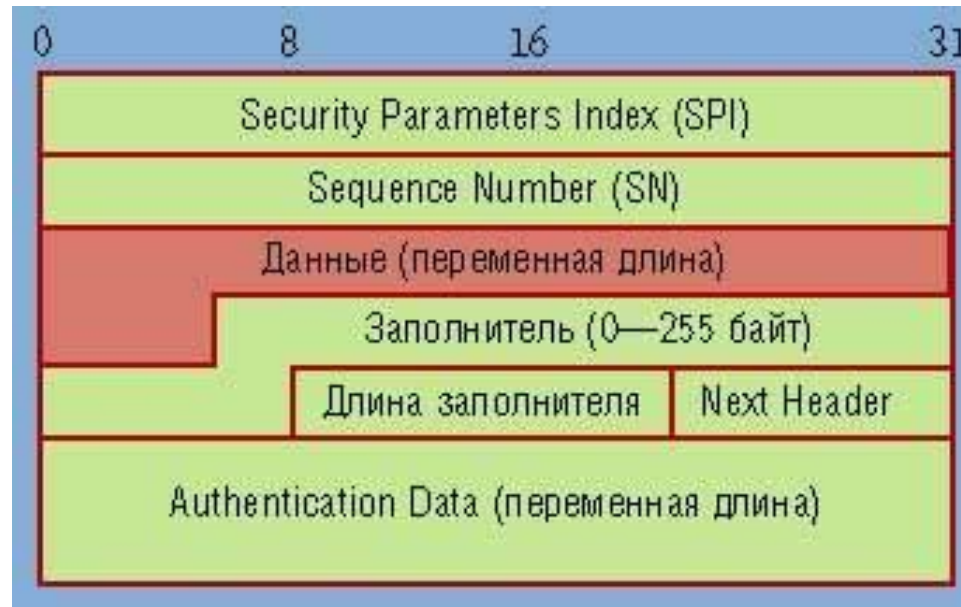
Структура заголовка протокола ESP.
