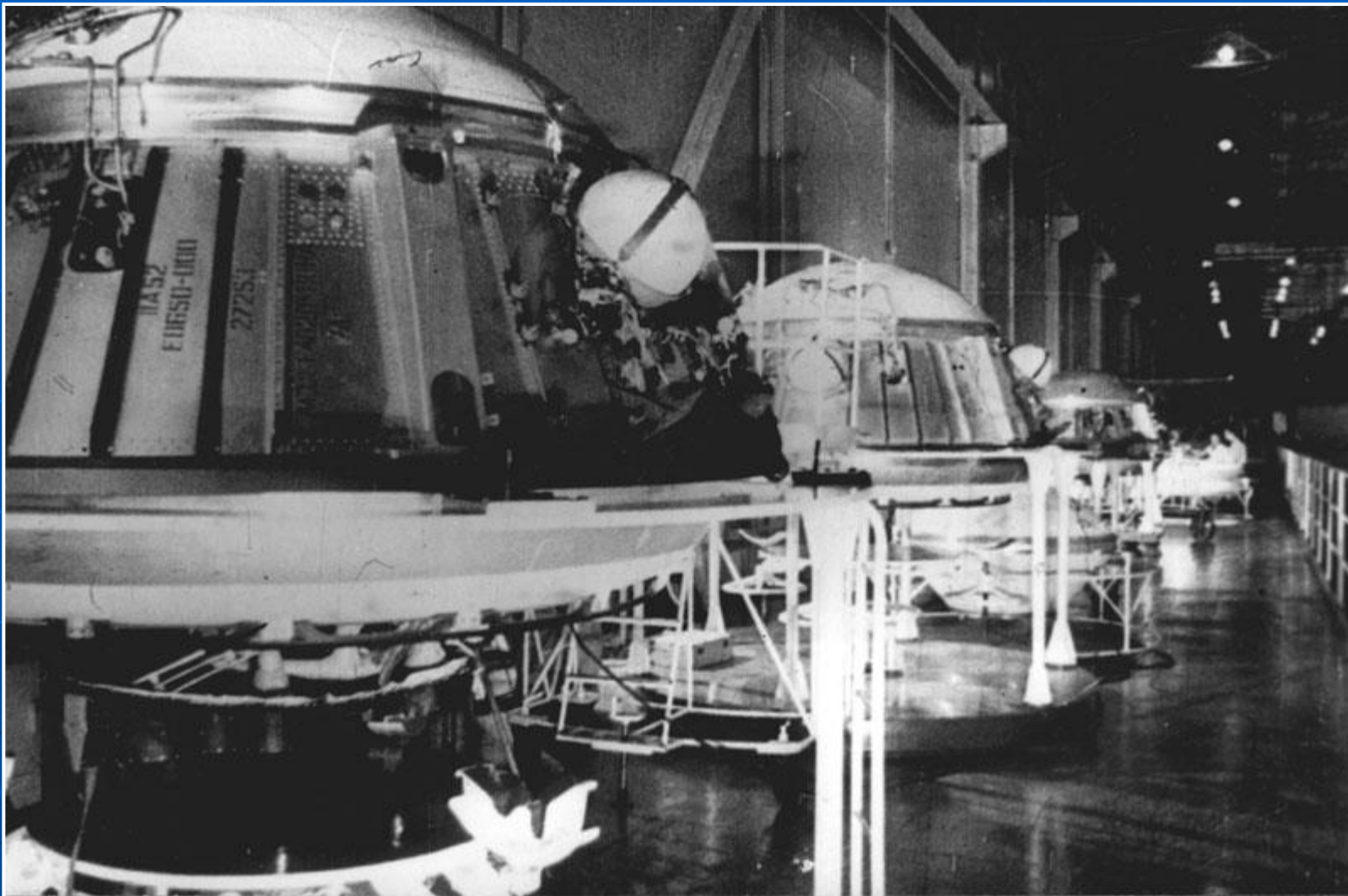
Разработанные в КБ «Южное» ракетные блоки Е лунного корабля в цехе завода «Южмаш» Ракетні модулі Е місячного корабля, які розроблені в КБ «Південне», в цеху заводу „Південмаш”
