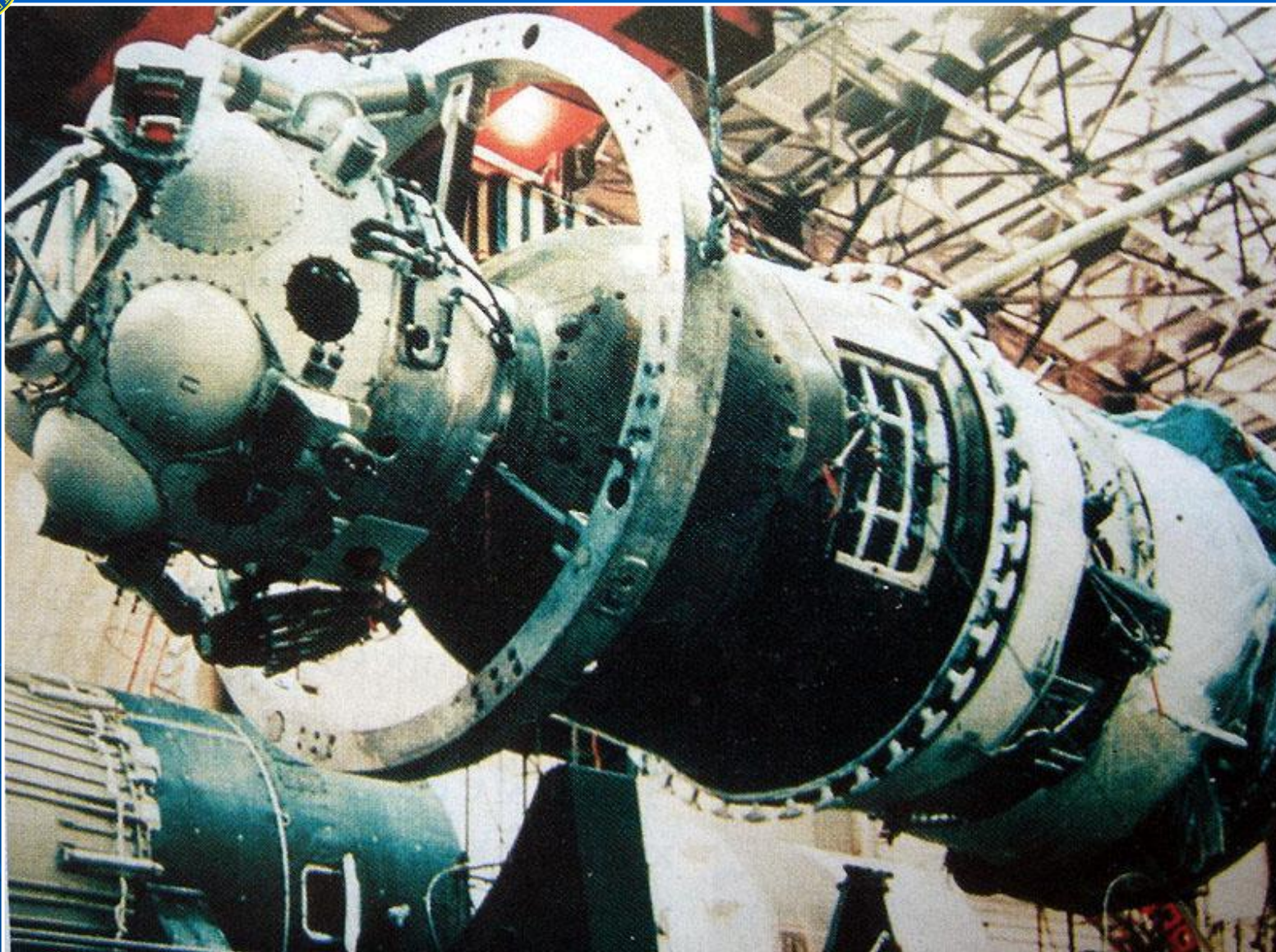
Лунный корабль С.П. Королева Місячний корабель С.П. Корольова
