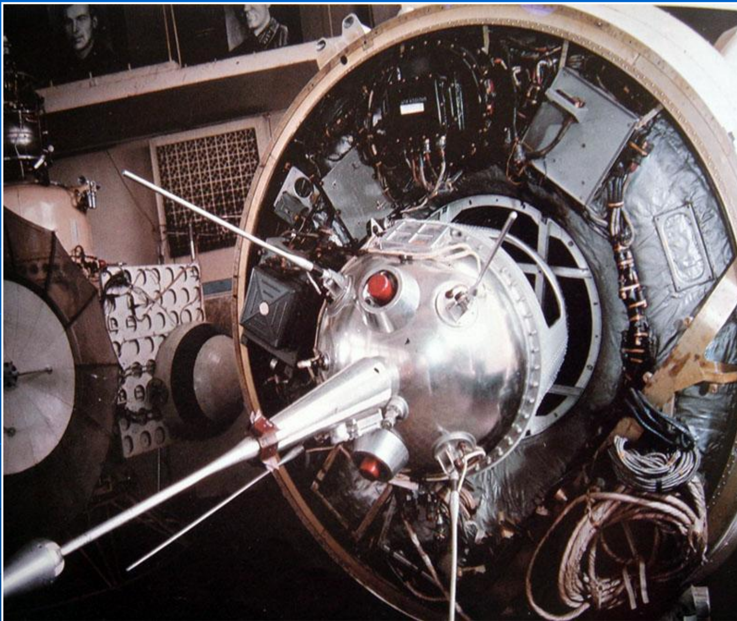
Автоматическая межпланетная станция «Луна-1»
