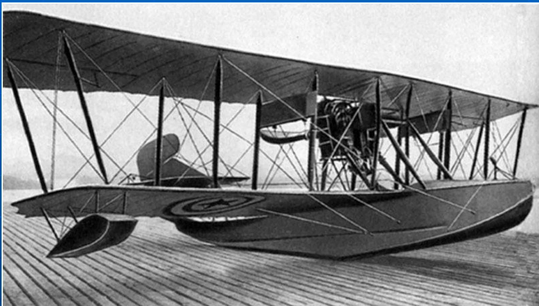
Летающая лодка М-9 конструкции Д.П. Григоровича, на которой осуществил свой первый полет С. Королев Літаючий човен М-9 конструкції Д.П. Григоровича, на якій здійснив свій перший політ С. Корольов
