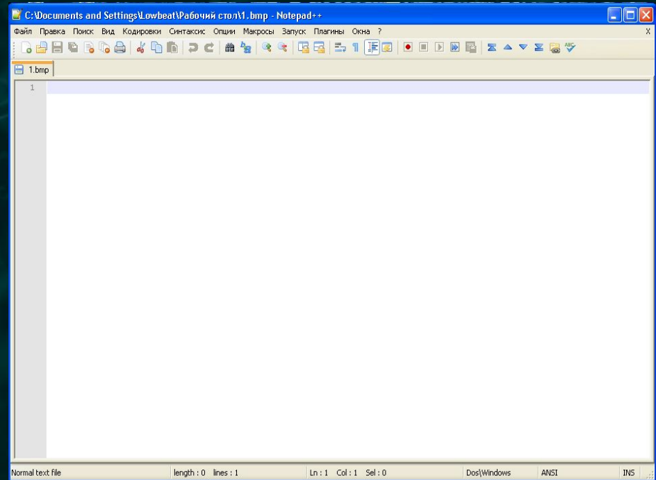
NotePad++
