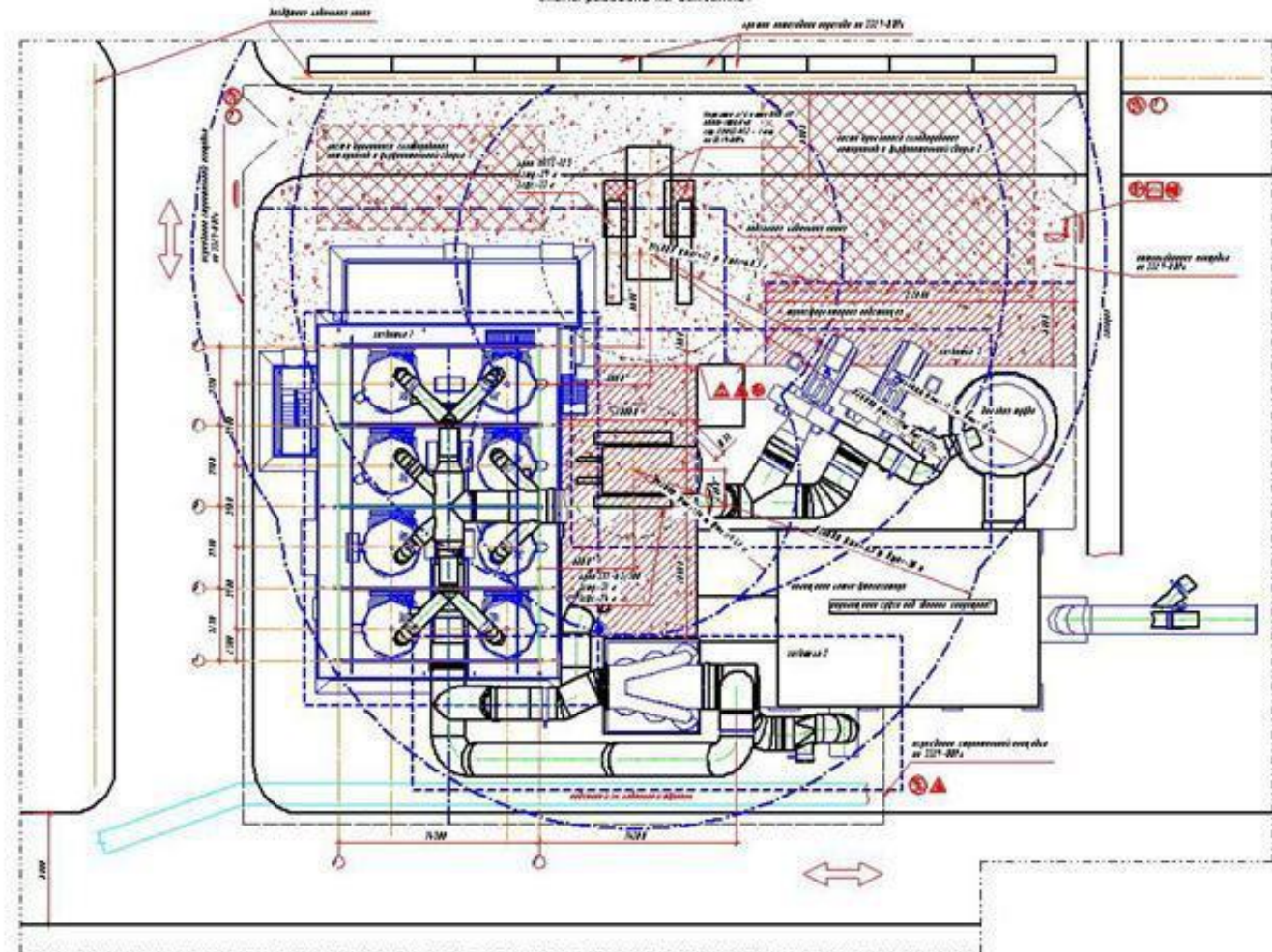
Ситуационный план № 11501. Схема разбивки на захватки
