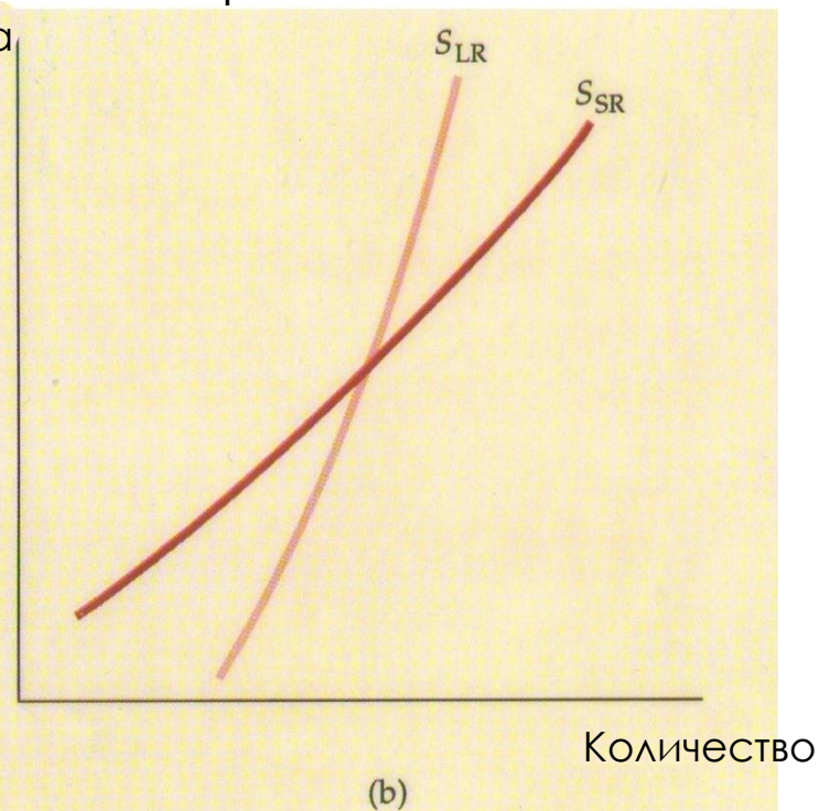
Вторичная медь
