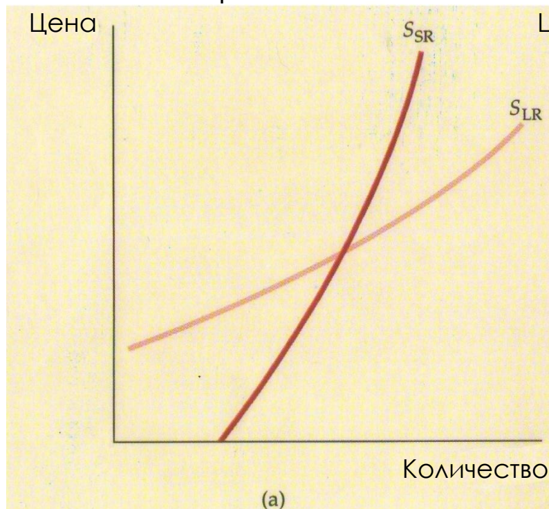
Первичная медь
