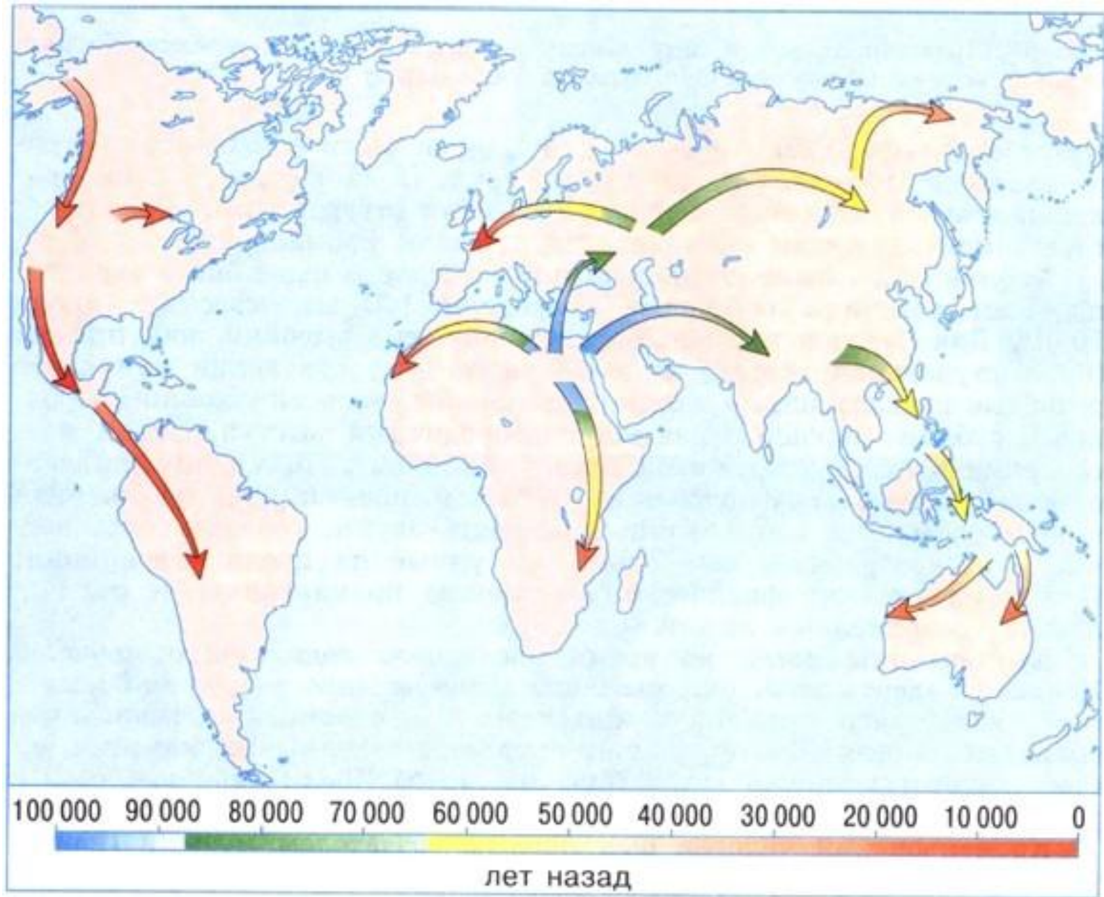
Расселение современного человека за последние 100 тыс. лет
