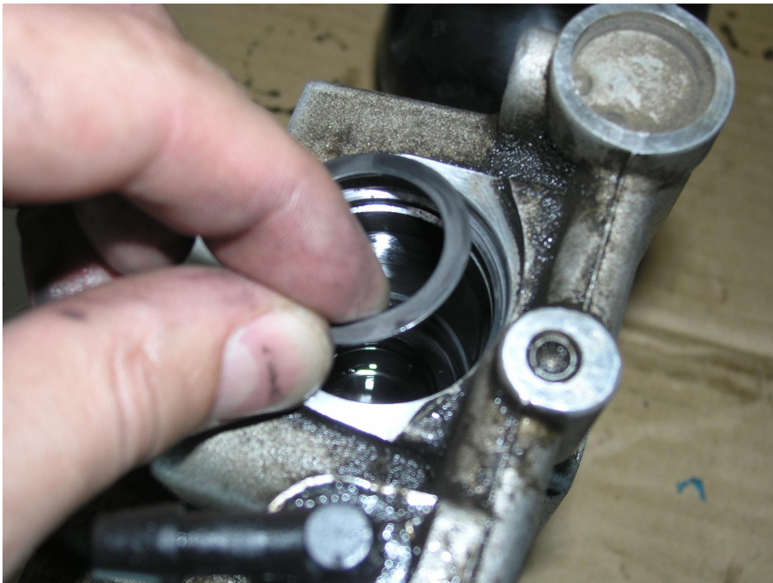
8. Пальцами извлекаем упорную шайбу манжеты рабочего цилиндра сцепления
