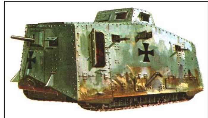
Первый танк Германии. Schwerer Kampfwagen A7V Длина - 8 м, ширина – 3,2 м, высота 3,5 м, вес 32,5 т.
