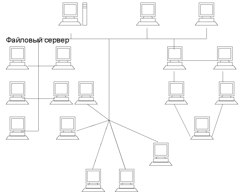
Древовидная структура ЛВС
