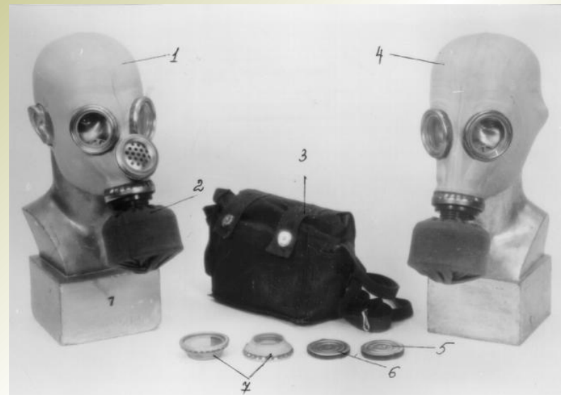
1 - шлем-маска ШМ-66 Му; 2 - фильтрующе-поглощающая коробка ЕО-62К в чехле; 3 - сумка; 4 - шлем-маска ШМ-62; 5 - непотепляющие пленки; 6 - мембраны переговорного устройства для ШМ-66 Му; 7 - накладные утеплительные манжеты
