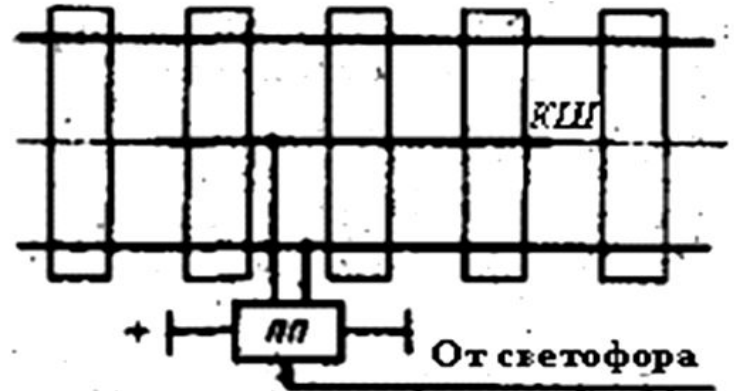
Электроконтактное устройство АЛСТ.
