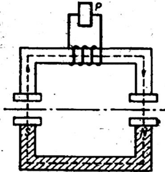
Схема АЛСТ индуктивного типа.
