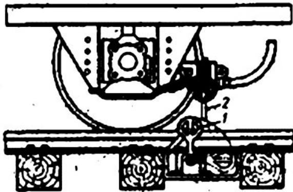
Механический датчик системы АЛСТ.
