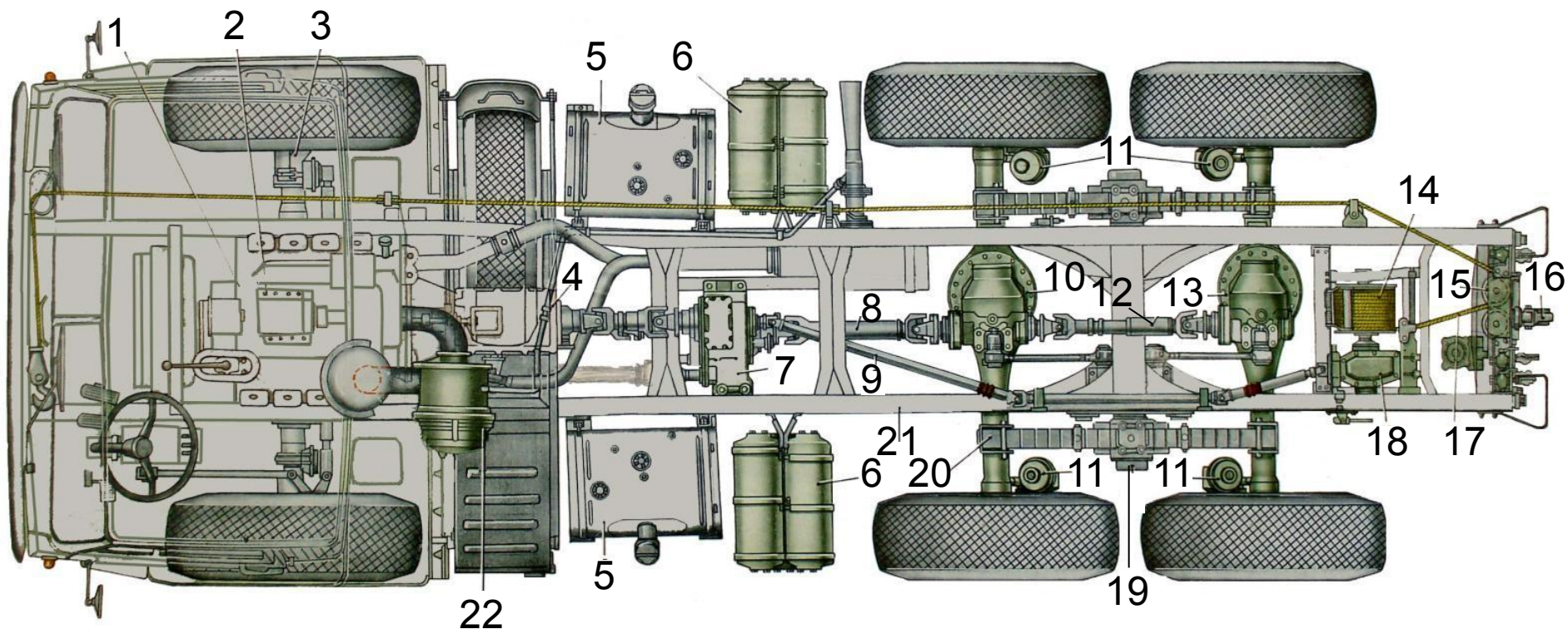
Общее вид автомобиля КамАЗ-4310
