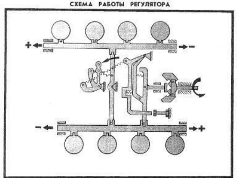
СХЕМА РАБОТЫ РЕГУЛЯТОРА
