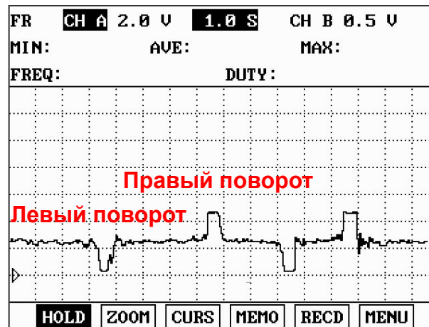
Выходной сигнал Yaw Rate sensor
