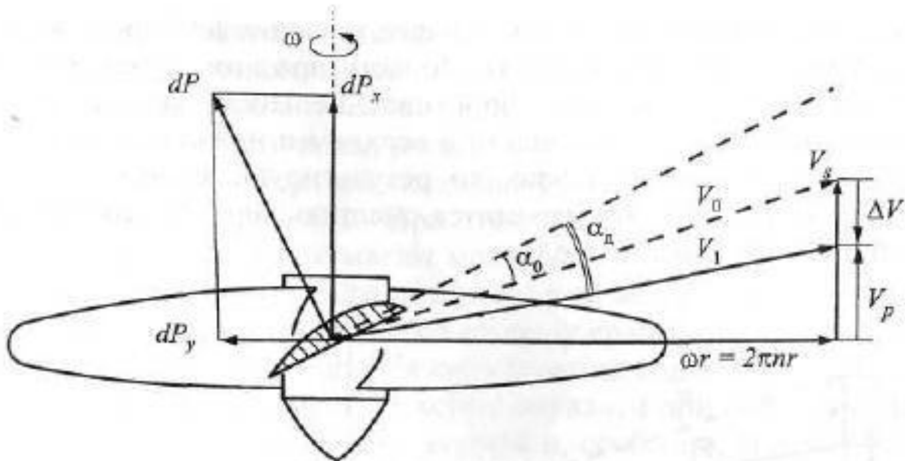
Рис. 1.9. Работа элемента лопасти вращающегося вперед гребного винта при движении судна передним ходом
