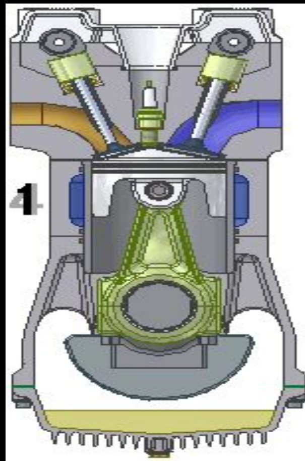
4-тактный двигатель
