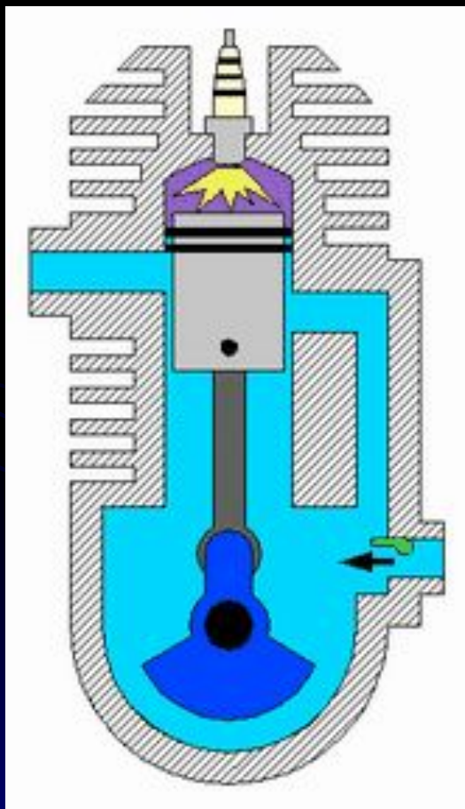
2-тактный двигатель
