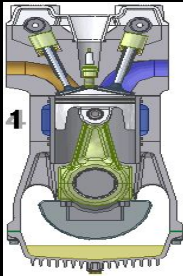
4-тактный двигатель
