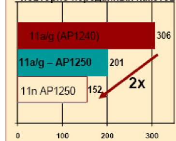
Среднее число повторно переданных пакетов
